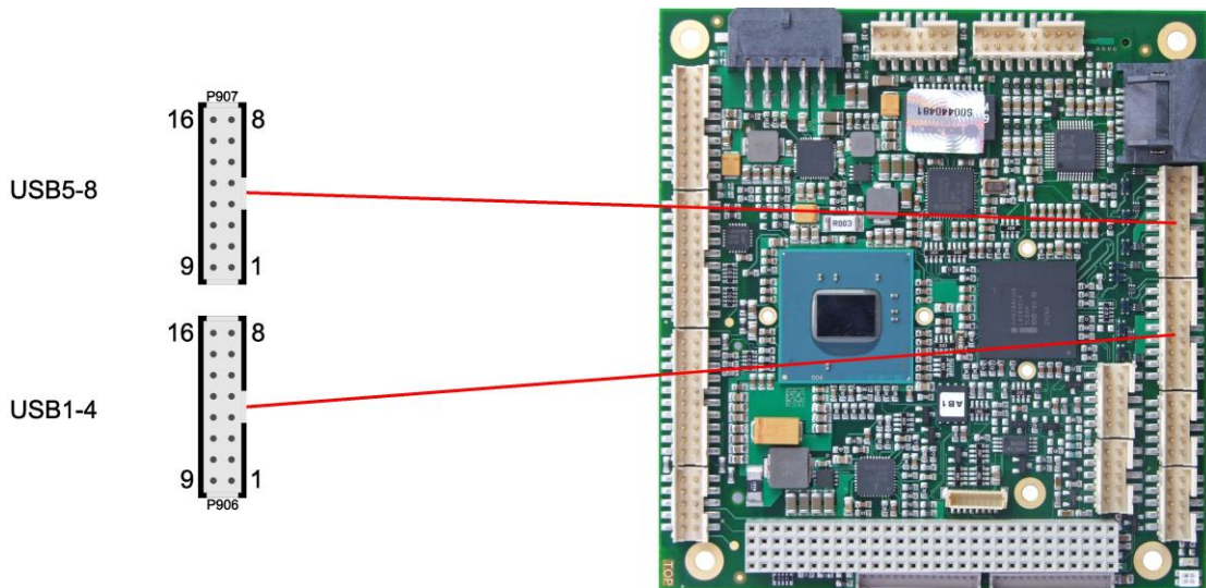
Pinbelegung USB 1-4:
